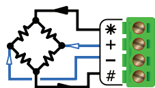
Voltage bridge (+ / #)
