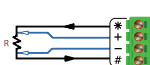
Platinum RTD (4 wire)
