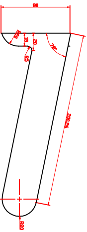
右视图
