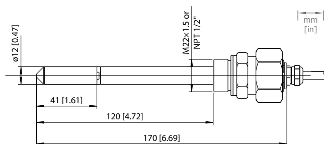
HMP374 dimensions
